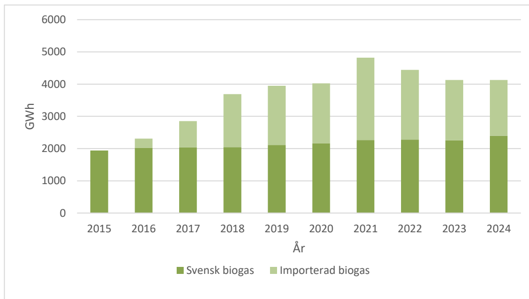
Figur S 1 Total biogasanvändning (GWh) i Sverige år 2015–2024, inklusive nettoimport via gasnät och flytande biogas (LBG).
