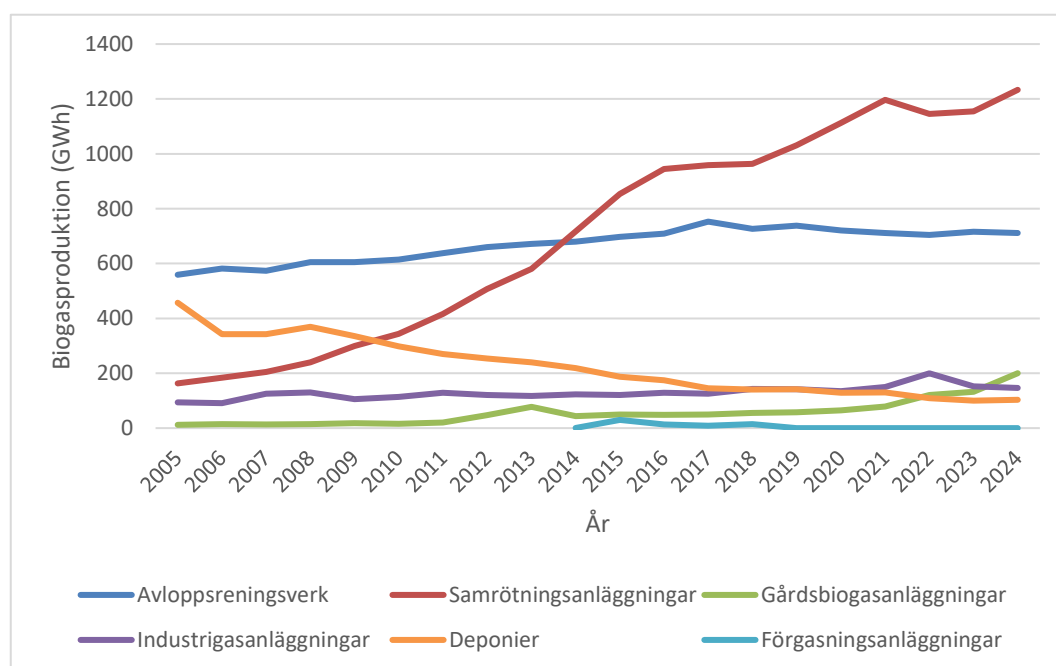
Figur 4 Utveckling av biogasproduktionen i Sverige per anläggningstyp, år 2005–2024.
