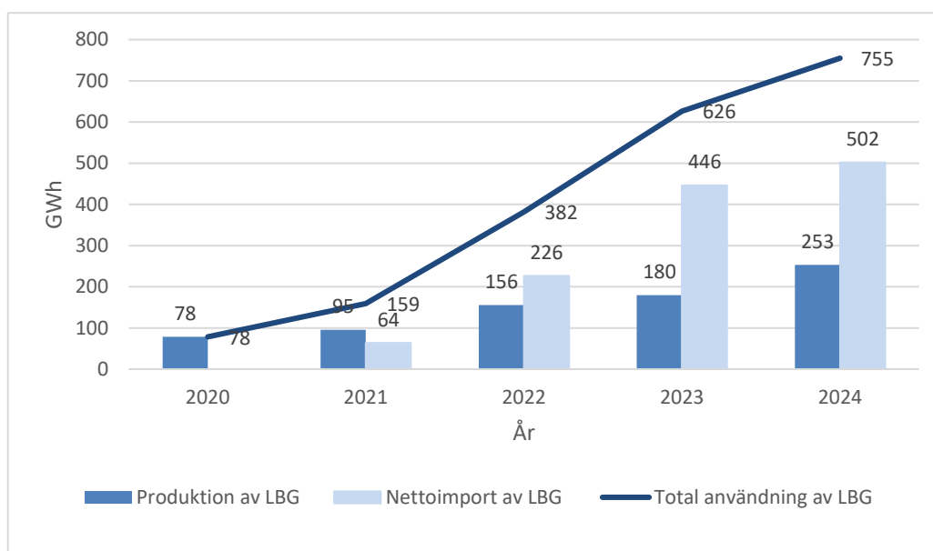
Figur 12 Produktion, nettoimport och total användning av flytande biogas (LBG) i Sverige, år 2020–2024.
