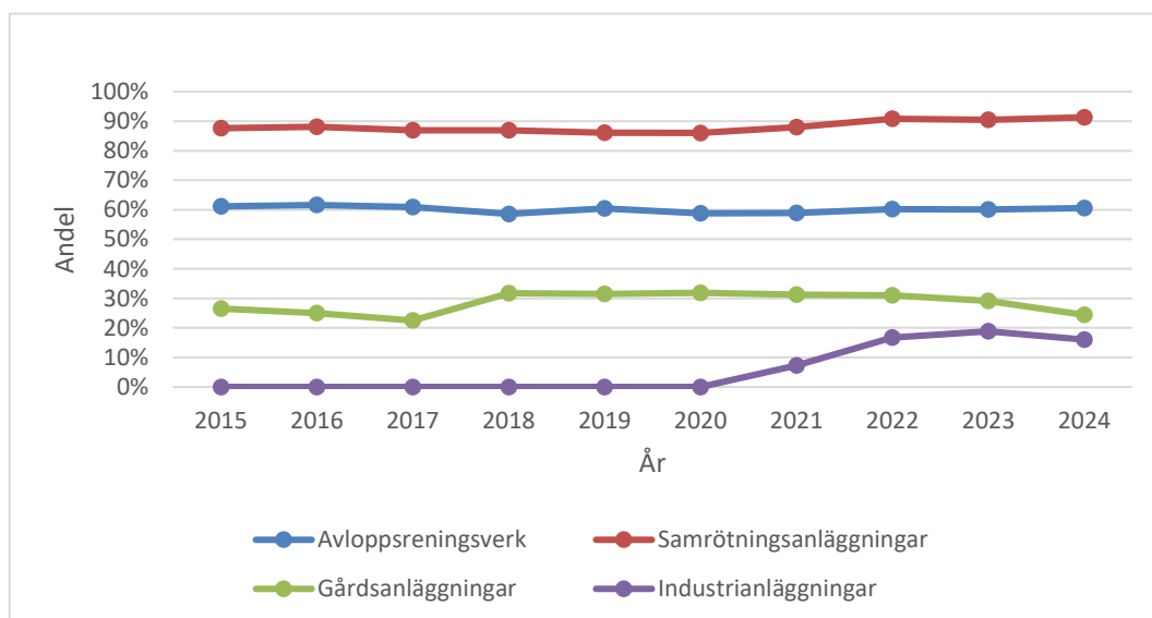
Figur 7 Andel biogas (%) som uppgraderas per anläggningstyp, år 2015–2024.
