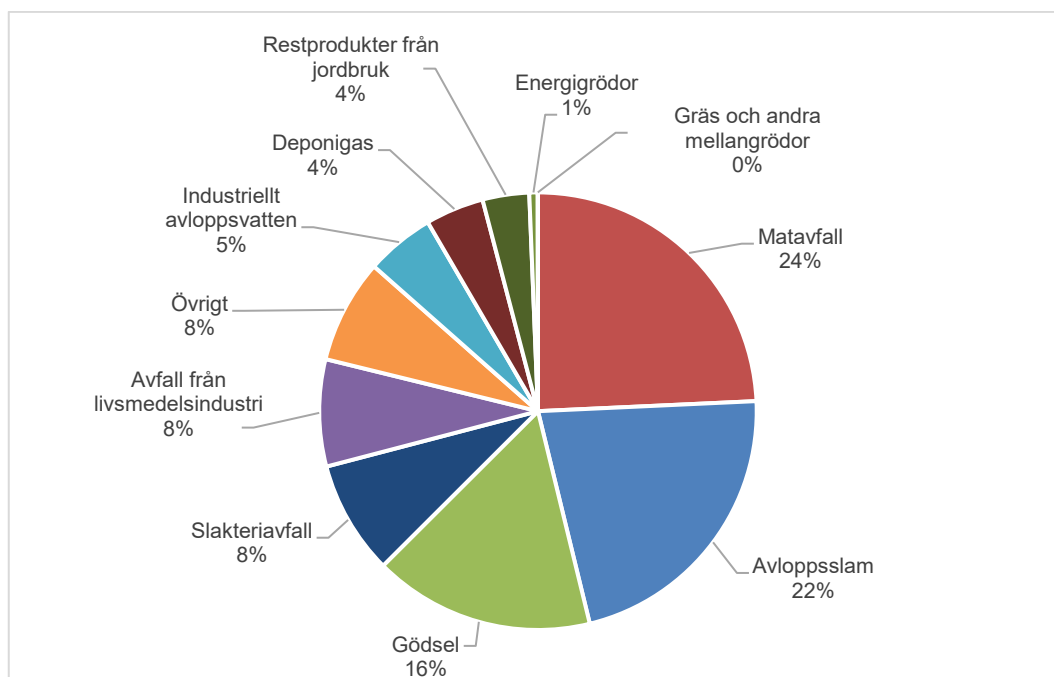
Figur 13 Andel producerad biogas (inklusive deponigas) från respektive substrattyp, beräknat med hänsyn till uppskattade biogasutbyten, år 2024. Observera att det är en uppskattning med stor osäkerhet. Använda mängder substrat (kton) framgår av Tabell 10 och antagna biogasutbyten framgår av Tabell 12.
