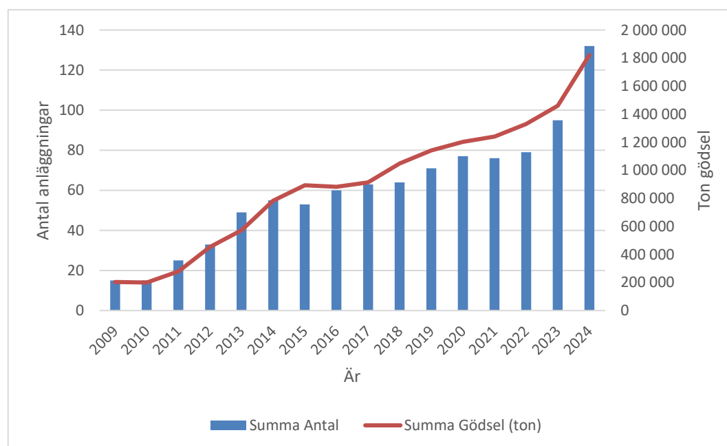
Figur 5 Mängd gödsel som rötas (ton) och antal anläggningar som producerar biogas från gödsel i Sverige, år 2009–2024.
